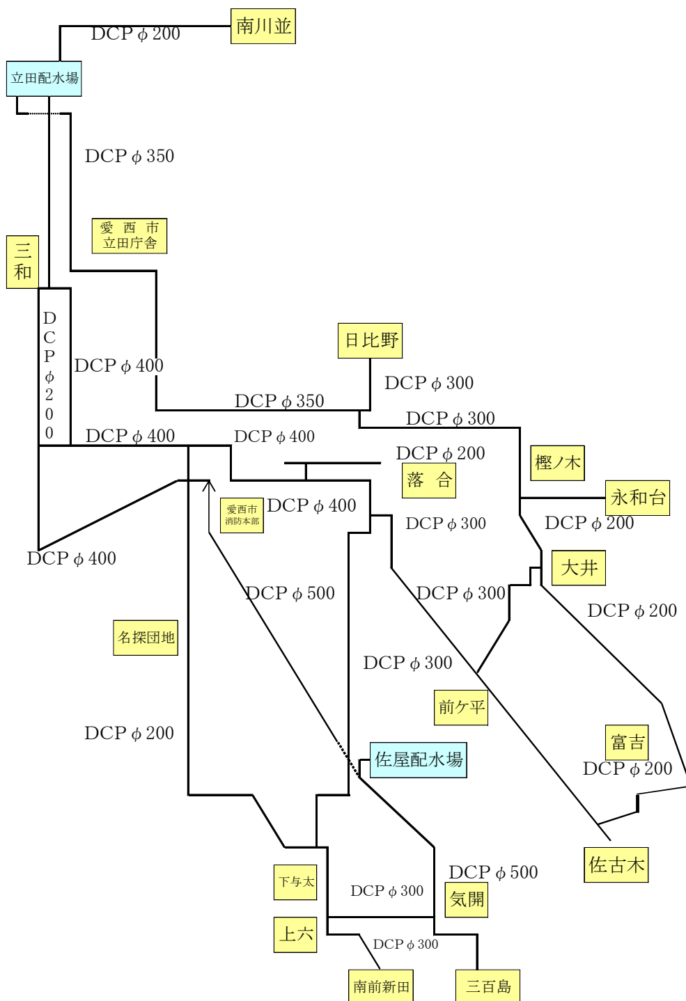
図 2-3 北部地区主要配管図
